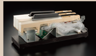
▲PHAⅡアイボリー・フィール鍵盤(エスケープメント付き)
